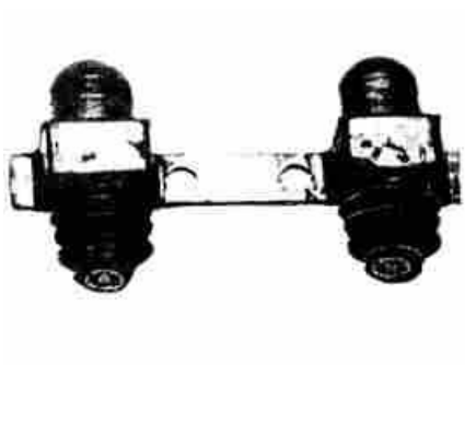
1069, SOPORTE TIRANTE PALANCA CAMBIOS FIAT DUNA-UNO (COMPLETO), GACRI-MILLGOM
