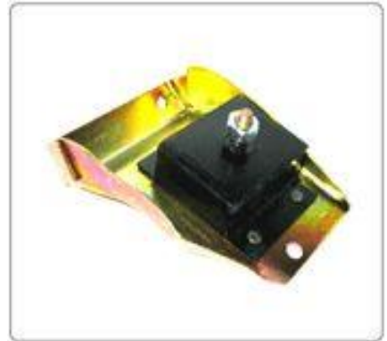
1030, SOPORTE MOTOR IZQUIERDO RENAULT 4S-6, GACRI-MILLGOM
